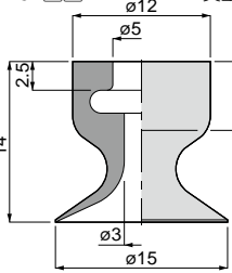
VP30L 5 6 質量：4.3g
