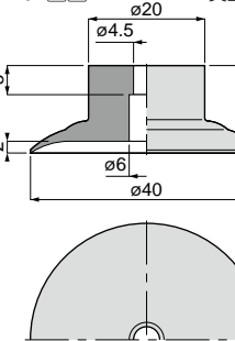
VP40L 5 6 質量：8.6g
