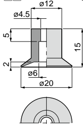
VP20L 5 6 質量：2g
