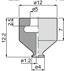
VP10L 5 6 質量：1.2g
