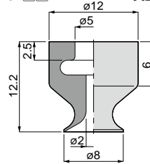
VP8L 5 6 質量：1.1g
