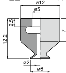
VP15L 5 6 質量：1.2g
