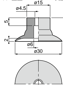
VP30L 5 6 質量：4.3g
