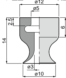
VP20L 5 6 質量：2g
